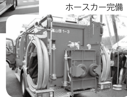
消防ポンプ車 (CD-1型)
