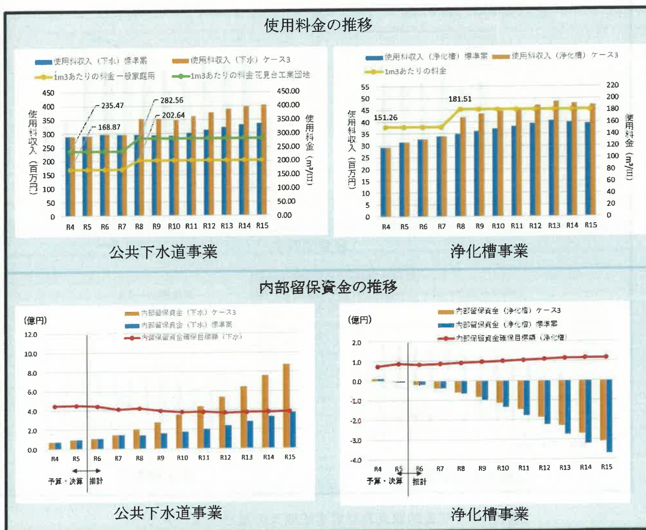
図 6-42 使用料金及び内部留保資金の推移（ケース 3）
