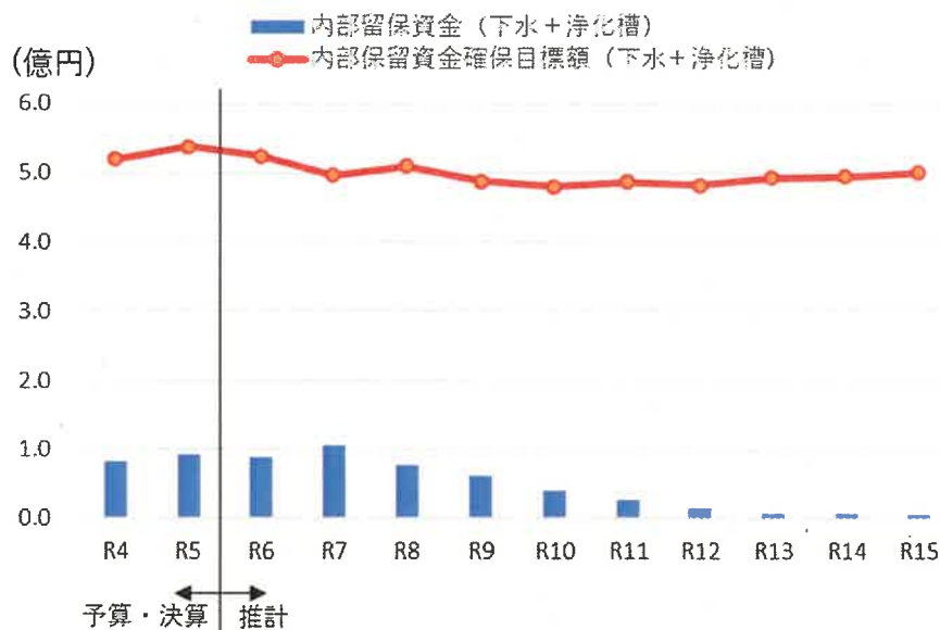
図 6-30 内部留保資金の見通し（公共下水道事業・浄化槽事業合算）
