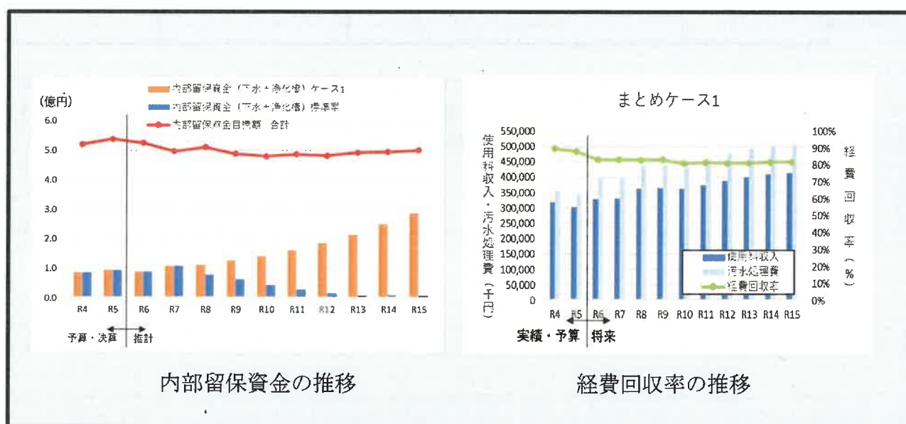
図 6-32 内部留保資金・経費回収率の推移（下水＋浄化槽）（ケース 1）
