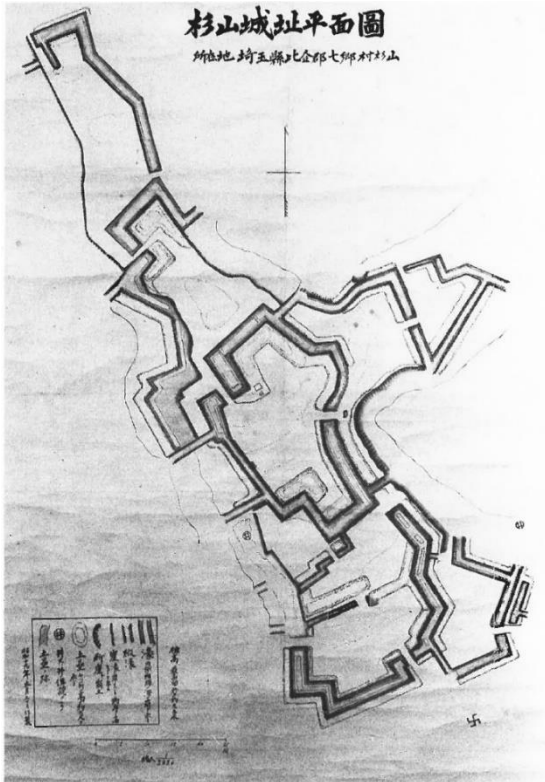
図6. 杉山城址平面図(金子,1944)
