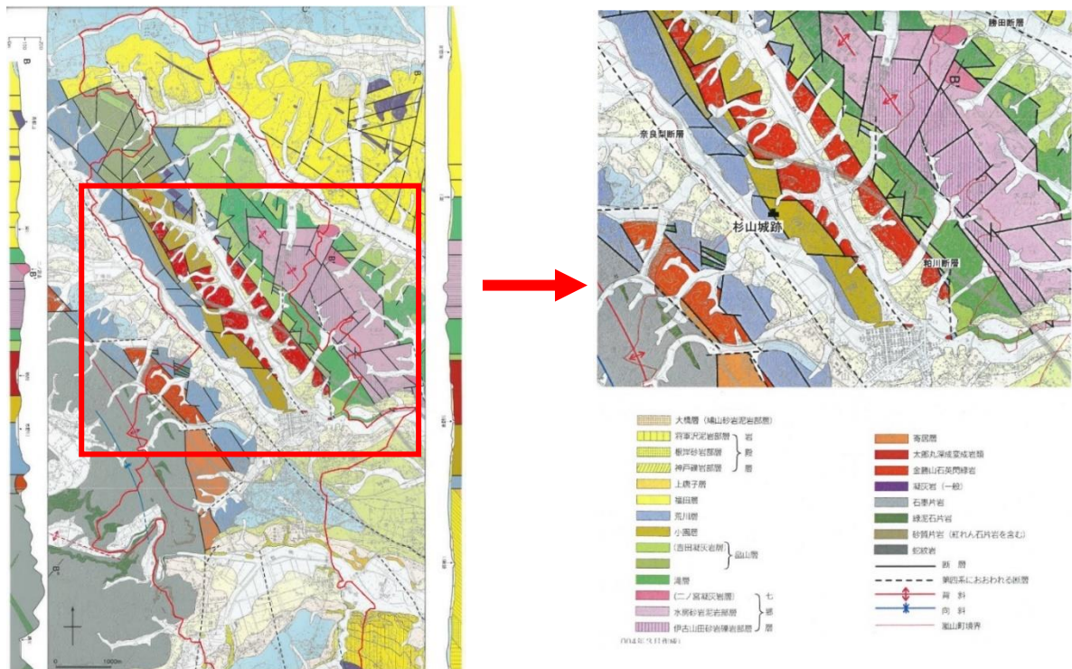
図 12. 嵐山町及び杉山城跡の周辺地域の表層地質図
